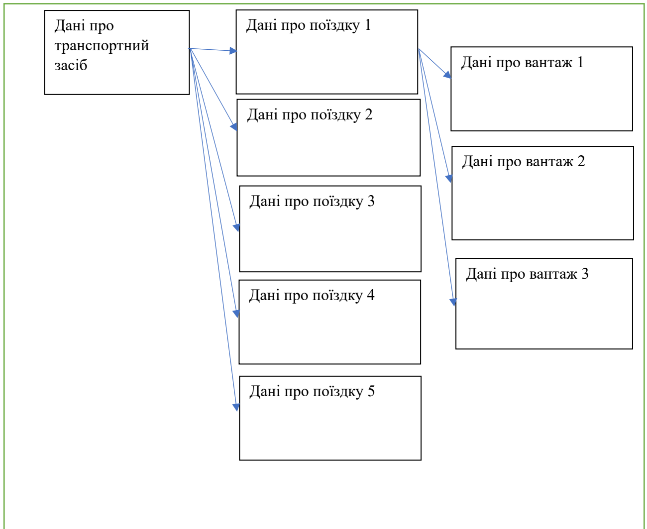
Рисунок 1. Структура даних
